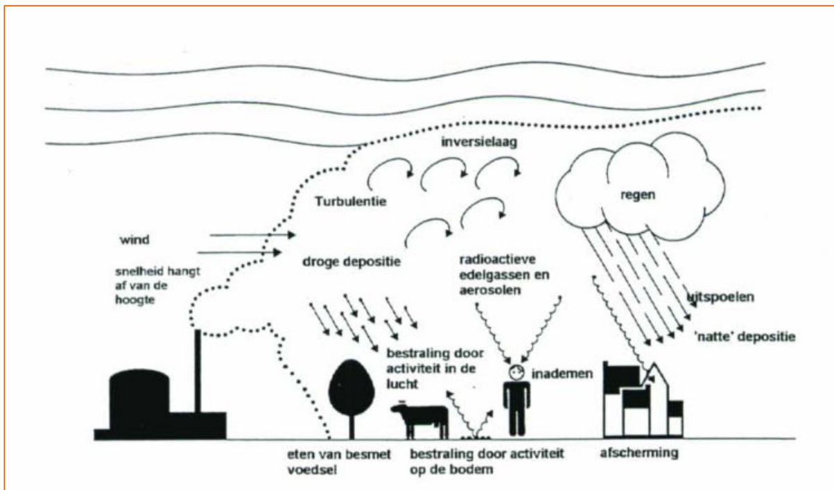
Figuur 1 Schematische weergave van de blootstellingsroutes voor radioactieve lozingen naar de lucht
