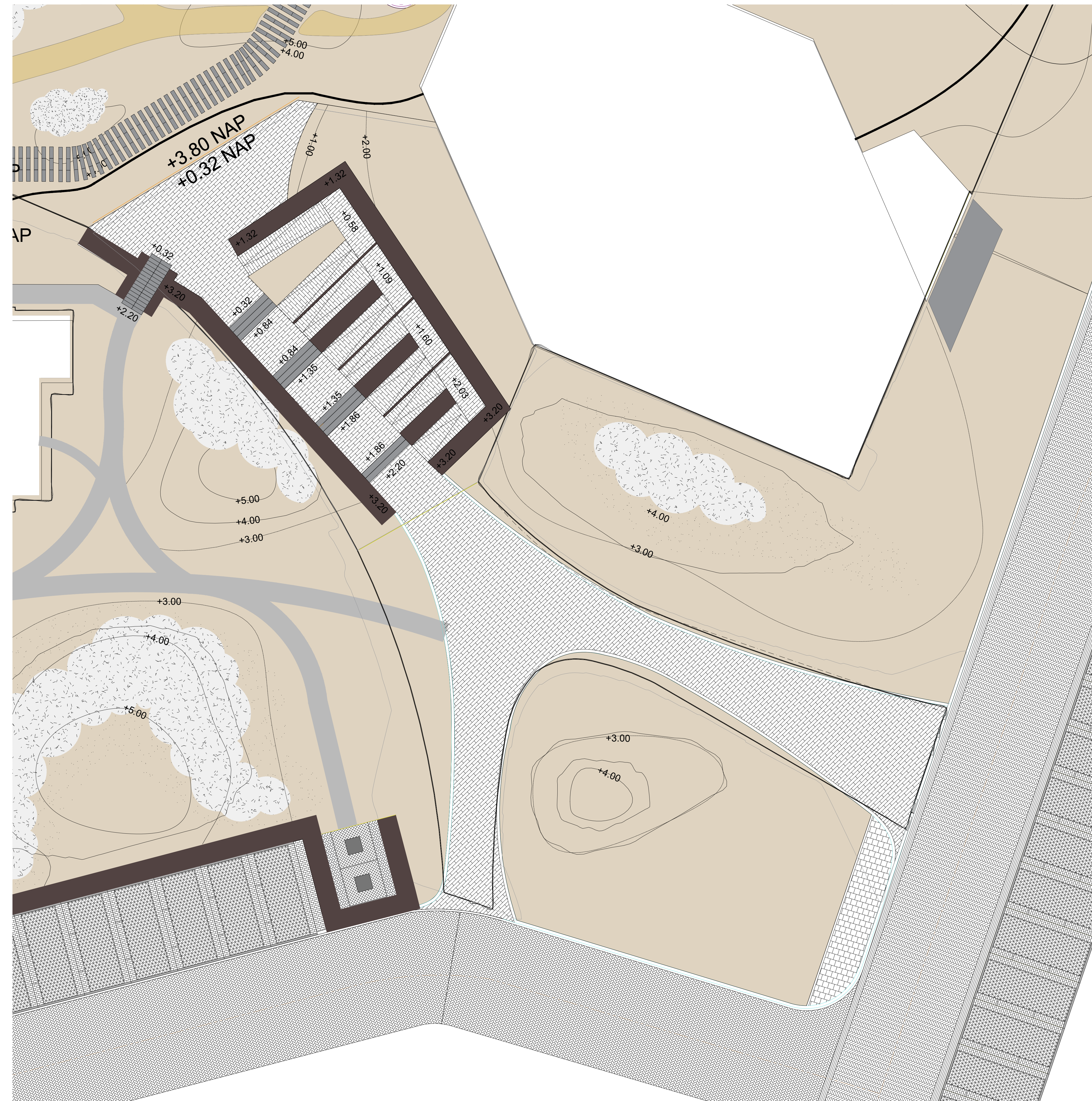
Detail trap/hellingsbaan 1:100
